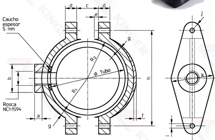
Abrazadera de arranque
