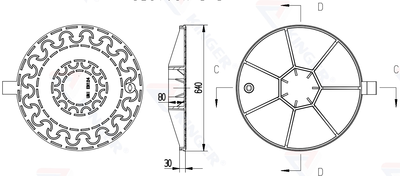
SECTION D-D
